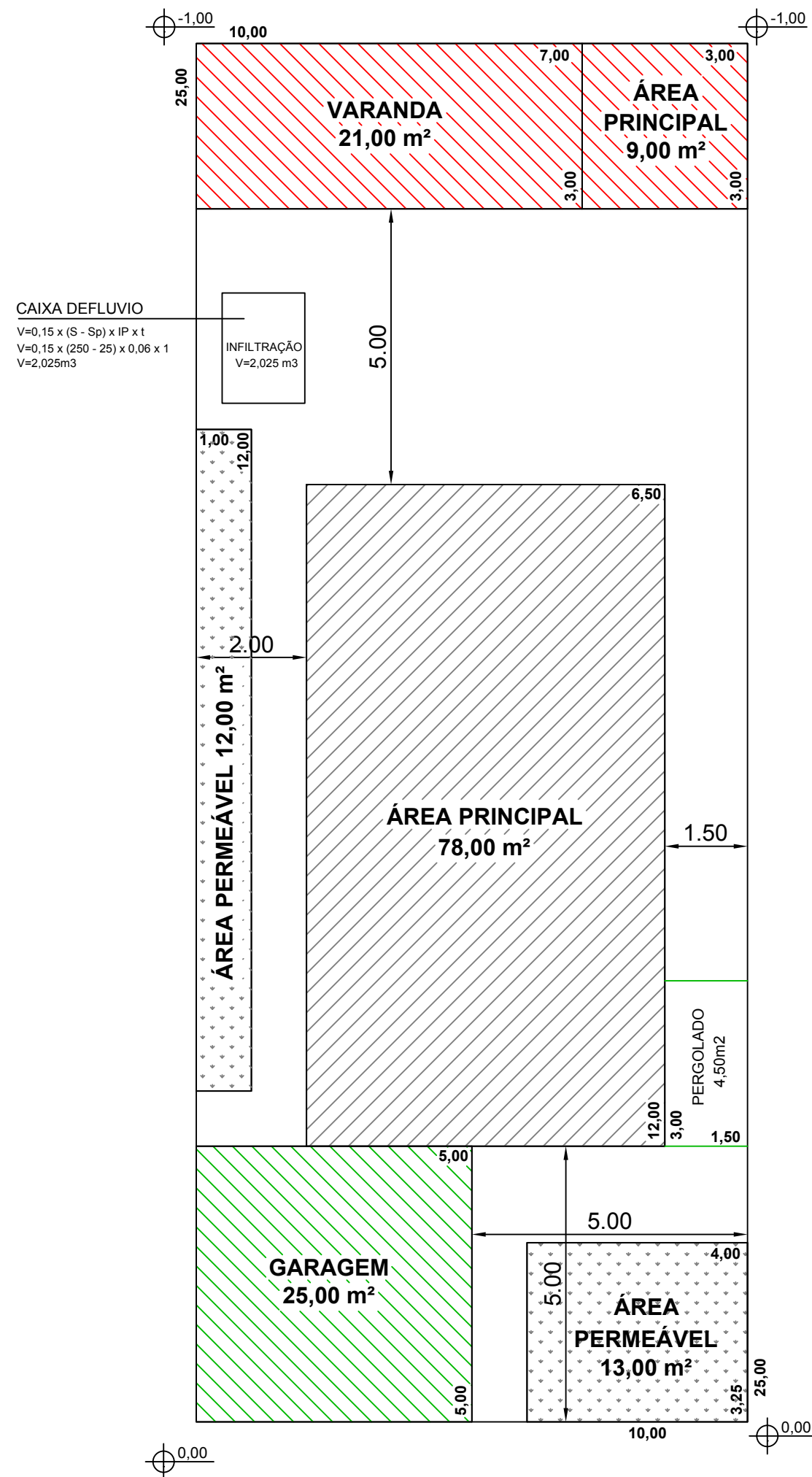
PAV. TERREO Escala 1:100
